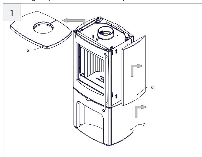
Retirer le couvercle (5)
