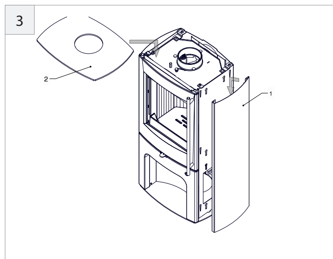
Le montage s'effectue dans l'ordre inverse.
