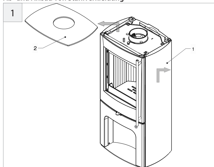
Abdeckung (2) abheben
