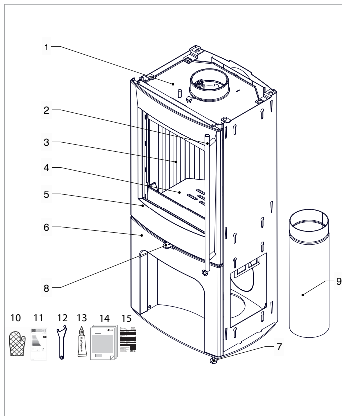
Contenu de la livraison de l'appareil de base
