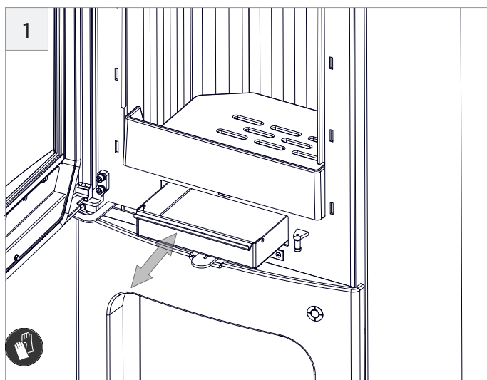
Entnahme und Einsetzen des Aschekastens.
