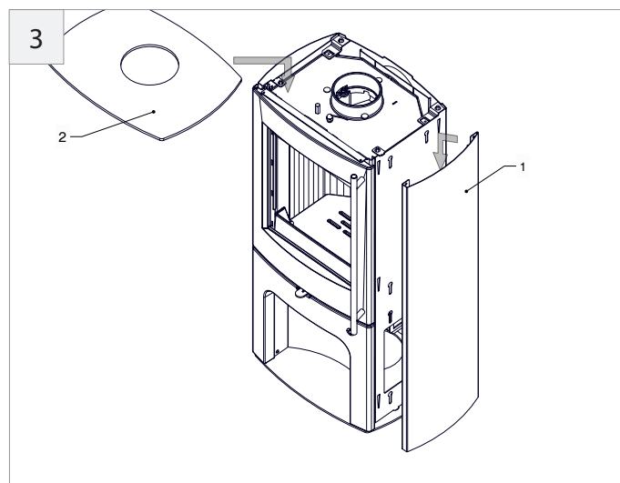
Der Anbau erfolgt in umgekehrter Reihenfolge.
