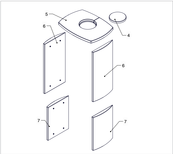
Übersicht der Naturstein Verkleidungselemente
