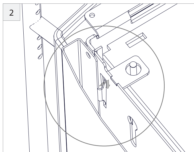
Schieben Sie das Seitenteil (1) nach oben, bis es in den Arretierungskeilen frei ist, und nehmen Sie es dann nach außen ab.
