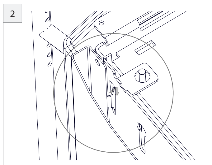
Faites glisser le panneau latéral (1) vers le haut jusqu'à ce qu'il se libère des cales de blocage, puis retirez-le vers l'extérieur.
