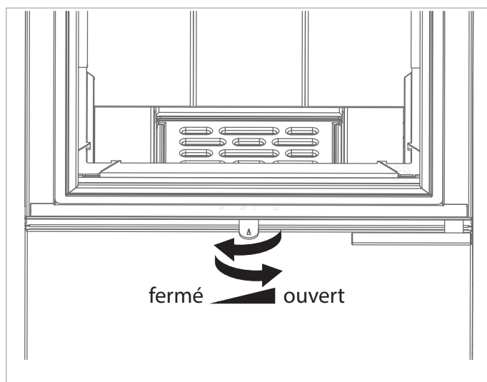
Fig. IV Réglage de l'air de combustion sur les poêles décoratifs équipés d'un levier rotatif (représentation schématique)
